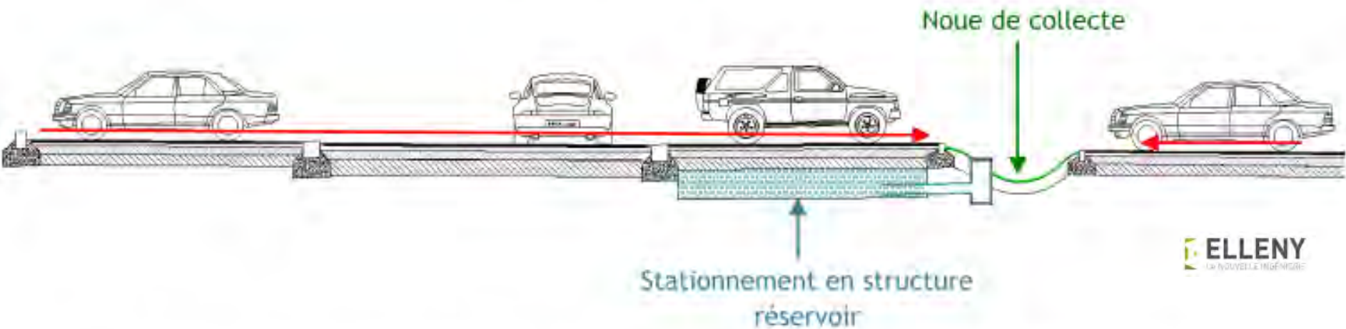
Coupe de principe de gestion des EP en structure réservoir sous stationnement
